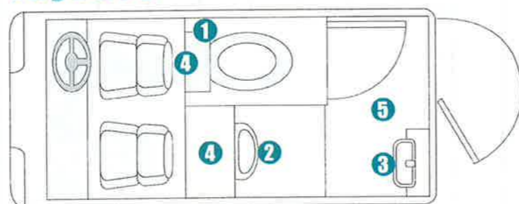
使いやすいように小便器、大便器、手洗い場の3つに分けたレイアウト。
