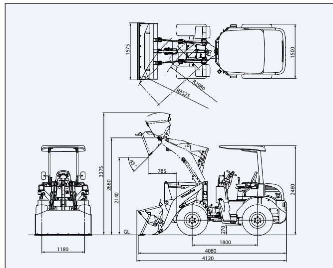
■ 外形図 /WA30-6
