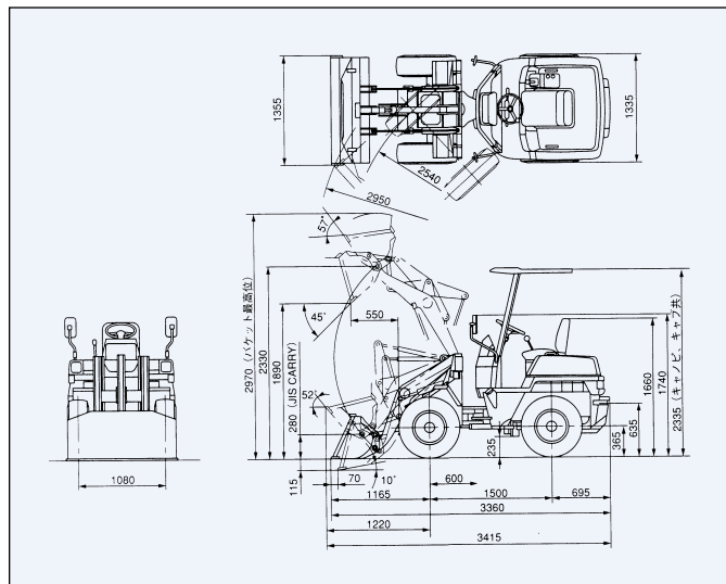
■ 外形図 /WA20-2E
