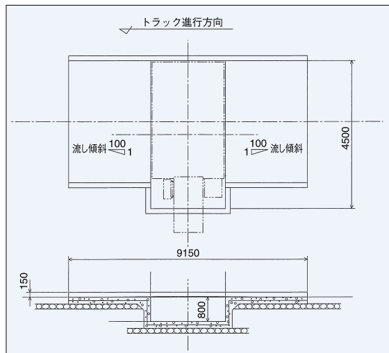
■ 据付寸法図 単位：mm
