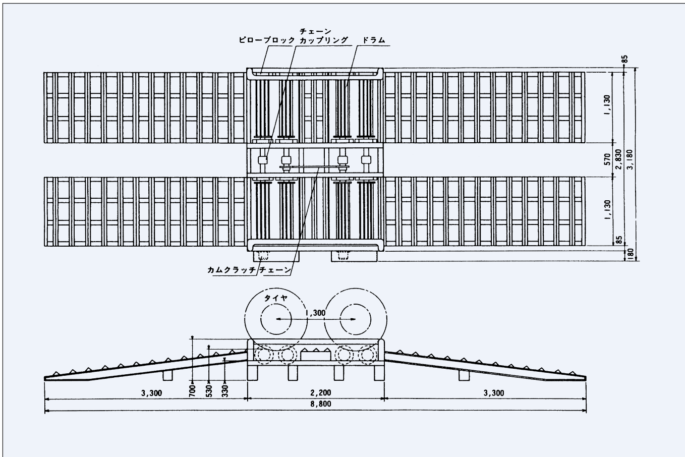
BD-II型（構造） もっともポピュラーなかさ上げ型
